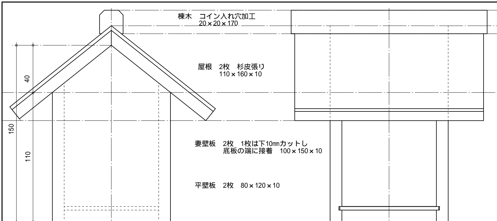
妻側立面図
